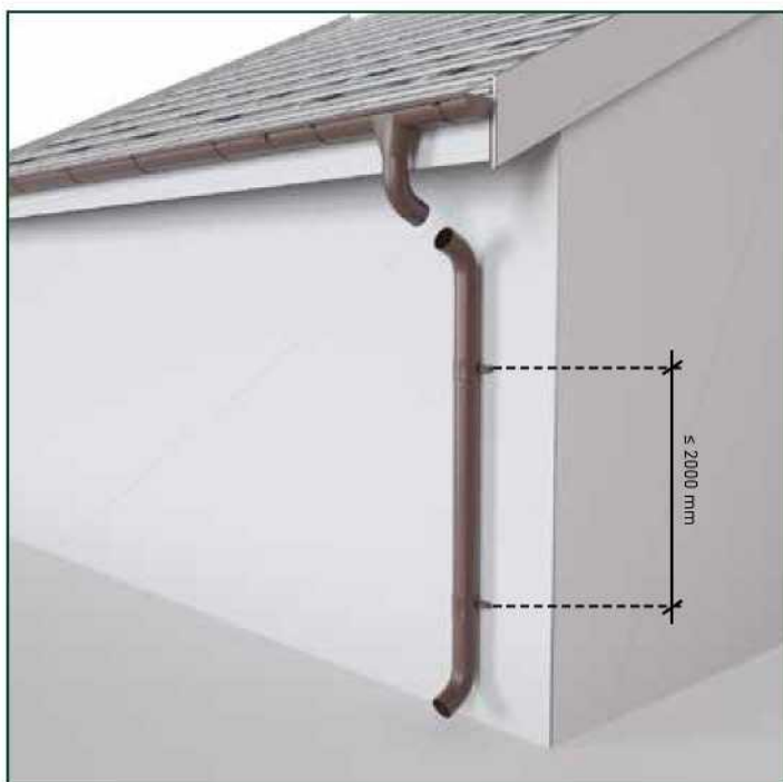
A konzolok közötti távolság nem haladhatja meg a 2000 mm-t.
